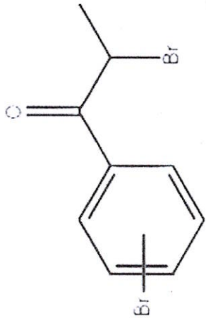
2-溴-溴苯丙酮
